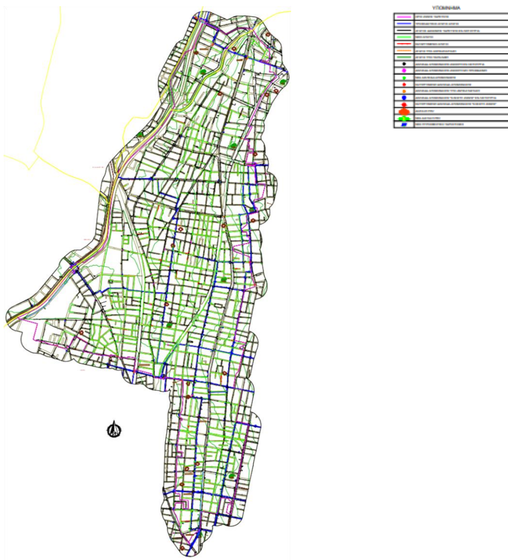
Εικόνα 10.: Γενική Διάταξη Έργων Πιεζομετρικής Ζώνης PRV Χαλεπά Σκοπέλου
